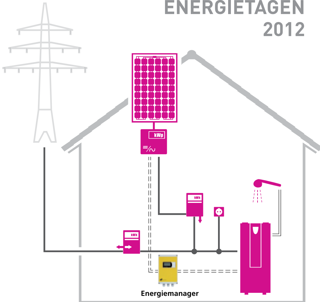
Das Cenpac plus verbindet Photovoltaikanlage, intelligenten Energiemanager und Warmwasser-Wärmepumpe.
